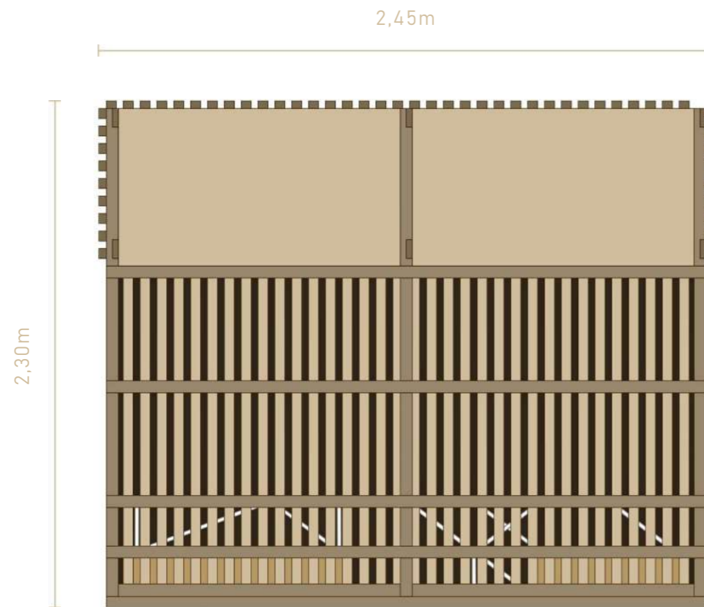
SPEISI Draufsicht
