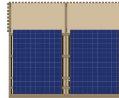
Module je 100cm x 132cm
